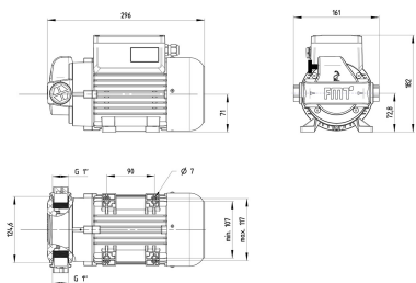
23301 Öl-Flügelzellenpumpe 30 l/min 230 V-1 AC-50 Hz-1,2 kW
